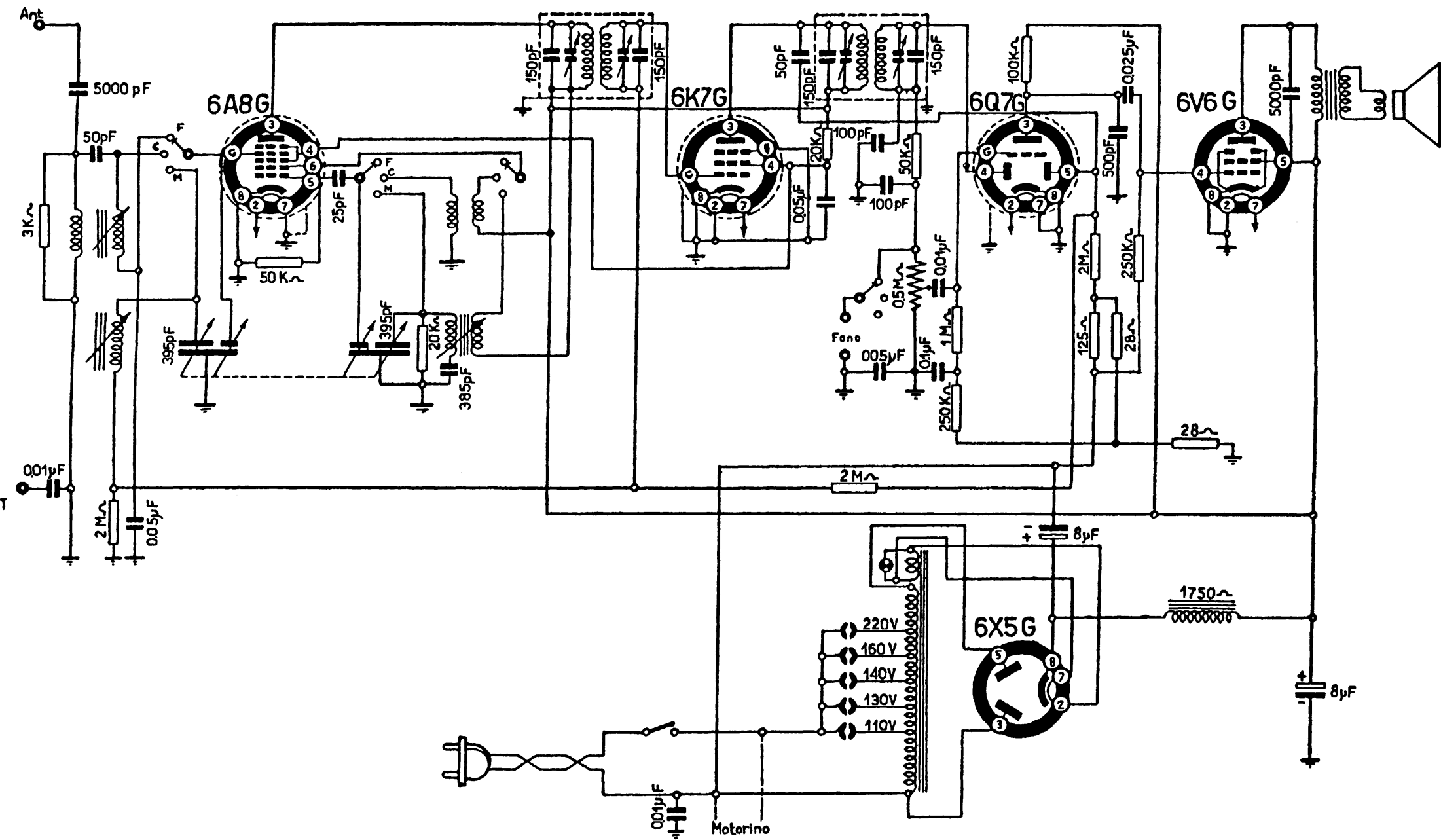
8 - CARISCH - MOD. CERVINO. Medie da 200 a 600 m, corte de 18 a 50 m. Schema come quello del mod. Sardegna e del mod. Lazio. Per il mod. Vesuvio v. Umbria, per mod. Bernina v. Mollise, per mod. Etna v. Calabria In « Radiolibro » 8ª ediz. MF: 465 kc/s.
